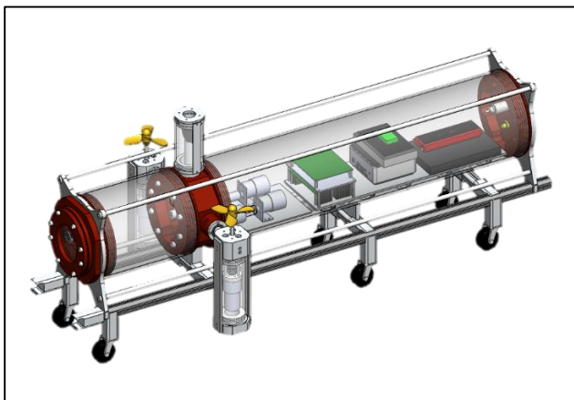
図 1 外観図
