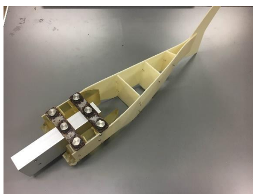
尾ひれ機構
