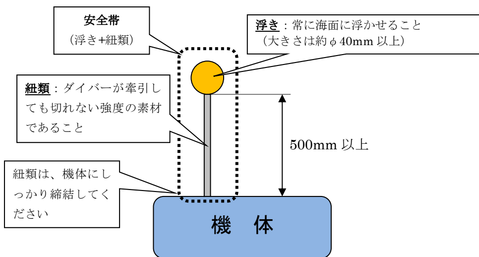
図 2-1-2 安全帯
