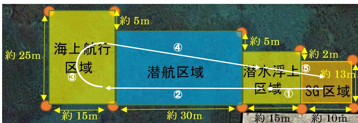
図 4-2-1 競技会場および競技コース航行例
