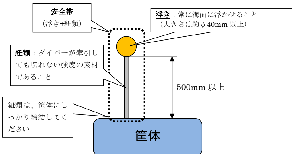
図 4-1-2 安全帯
